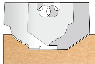
Scale -1:1 3510358+3510500
