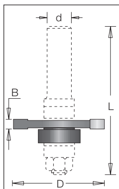
Arbor & Nut #190 004 3 L=67
