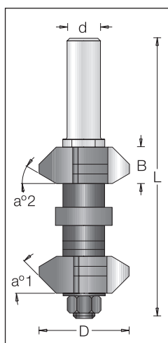
Arbor & Nut #190 011 9 L=108
