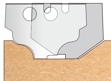
Scale -1:1 3510358+3510501
