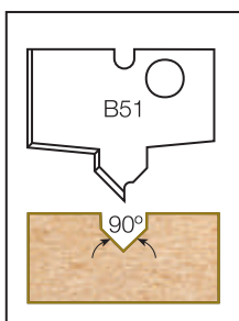
T.C. Blade
