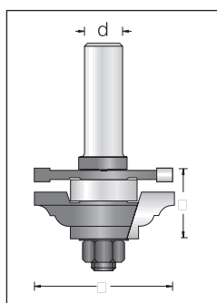
Arbor & Nut #190 004 5 L=70
