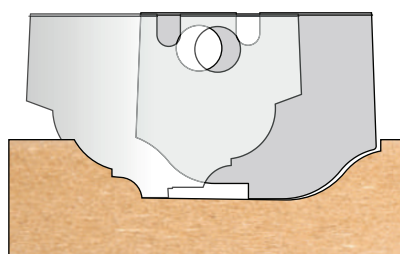
Scale -1:1 3510360+3510500
