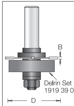
Spacer #192 050 0 0.05x16
